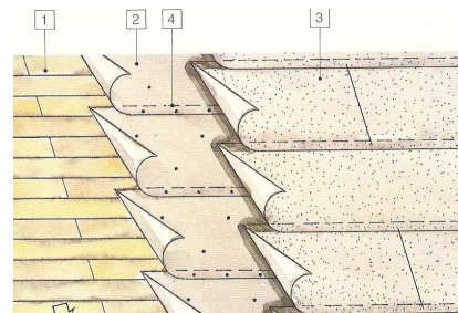
1. dřevěný podklad 2. první vrstva 3. druhá vrstva 4. mechanické kotvení
